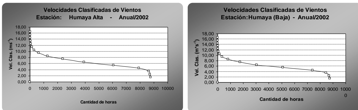
FIGURA Nº 3: Curva de velocidades clasificadas por rangos de 1 \text{ ms}^{-1} para el período de medición. Humaya Alta y Humaya de Abajo: Año 2002.
