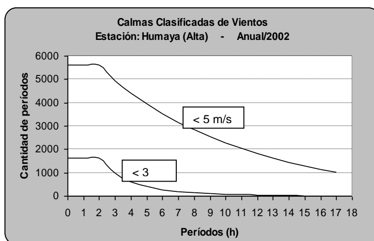
FIGURA Nº 4: Períodos de calmas, clasificados por horas de duración, donde la velocidad media horaria es inferior a 3 \text{ ms}^{-1} y a 5 \text{ ms}^{-1} , por ser consideradas límites para el arranque de las turbinas lentas y rápidas respectivamente. Humaya de Arriba: Año 2002. Dpto. Ambato – Catamarca.
