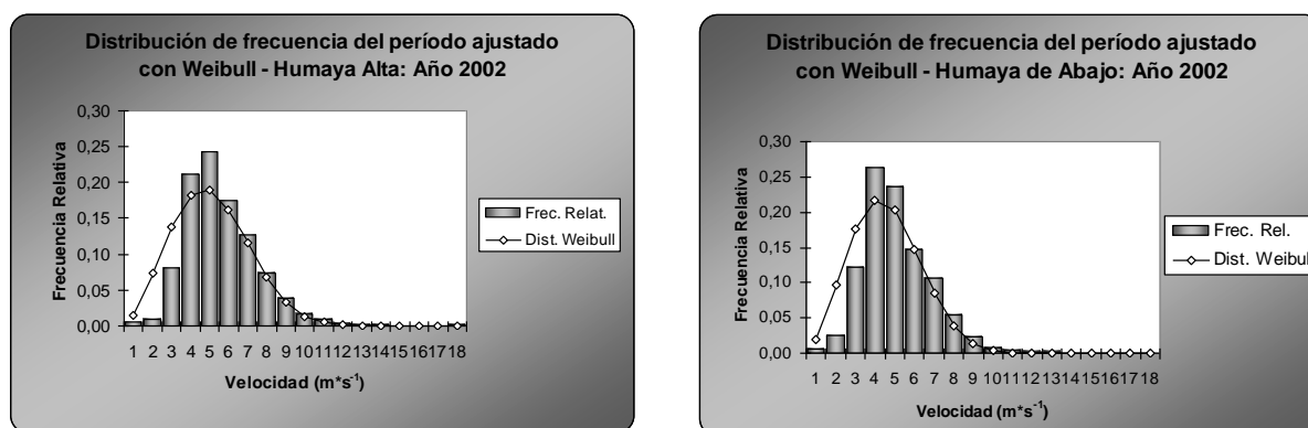
FIGURA N° 2: Histograma de Distribución de Frecuencia Relativa anual, ajustada matemáticamente con la función de Weibull II, para ambas estaciones registradoras. Humaya Alta y Humaya de Abajo – Año 2002.
