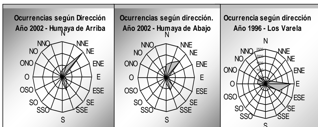
FIGURA N°5: Distribución de la frecuencia (ocurrencia) de dirección de viento según la rosa de los vientos, para cada una de las localizaciones: Humaya Alta y Humaya de Abajo. Año 2002; Los Varela: Año 1996.
