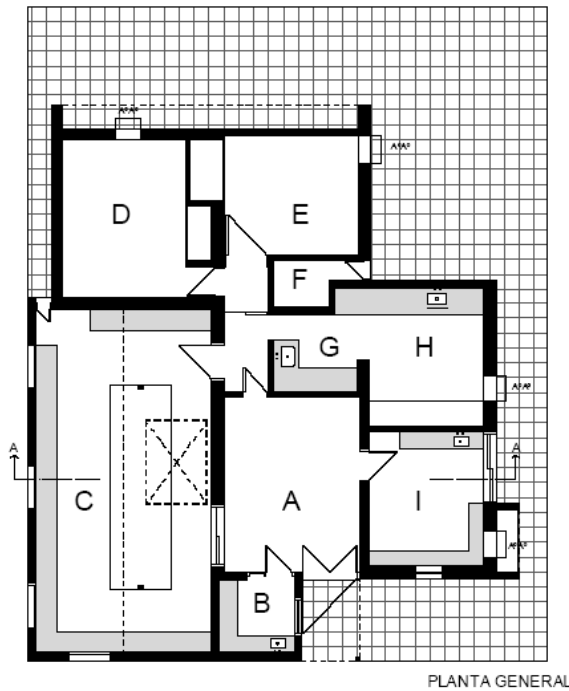
Figura 1. Planta general del centro experimental.
