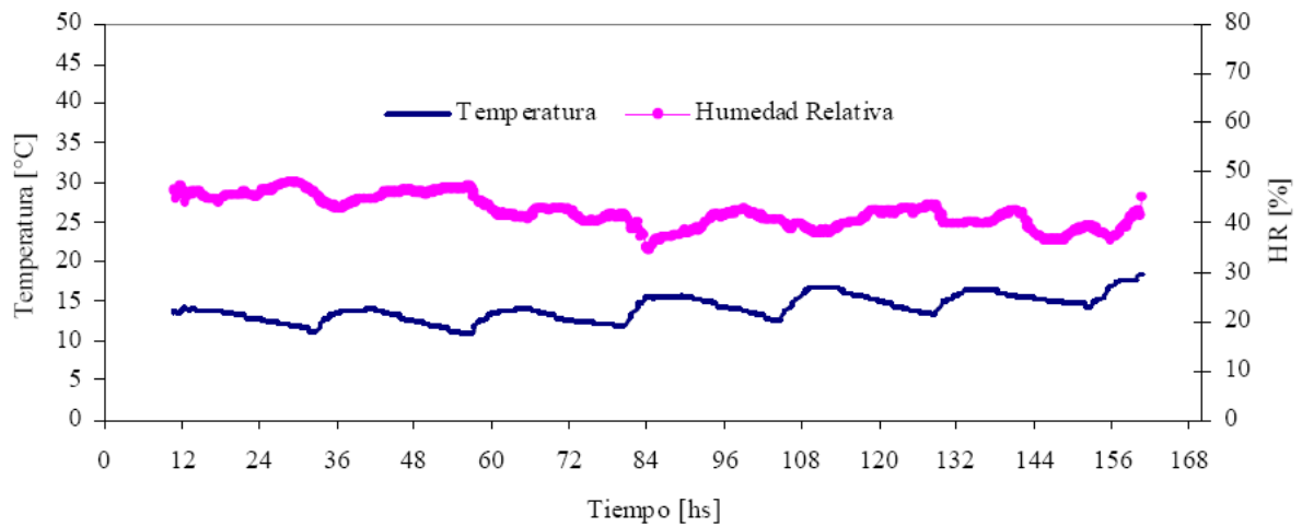
Fig. 15. Temperatura y humedad relativa en la sala de dosificación.
