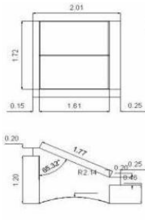
Fig. 8. Detalle del conjunto diseñado
