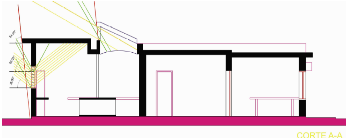
Figura 11: Corte del edificio con modificación e incorporación de sistemas de iluminación natural.
