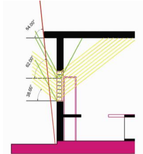
Fig. 6. Dibujo de rayos incidentes y redirección de la iluminación solar directa
