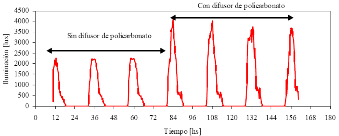
Fig. 13: Iluminación en la sala de dosificación
