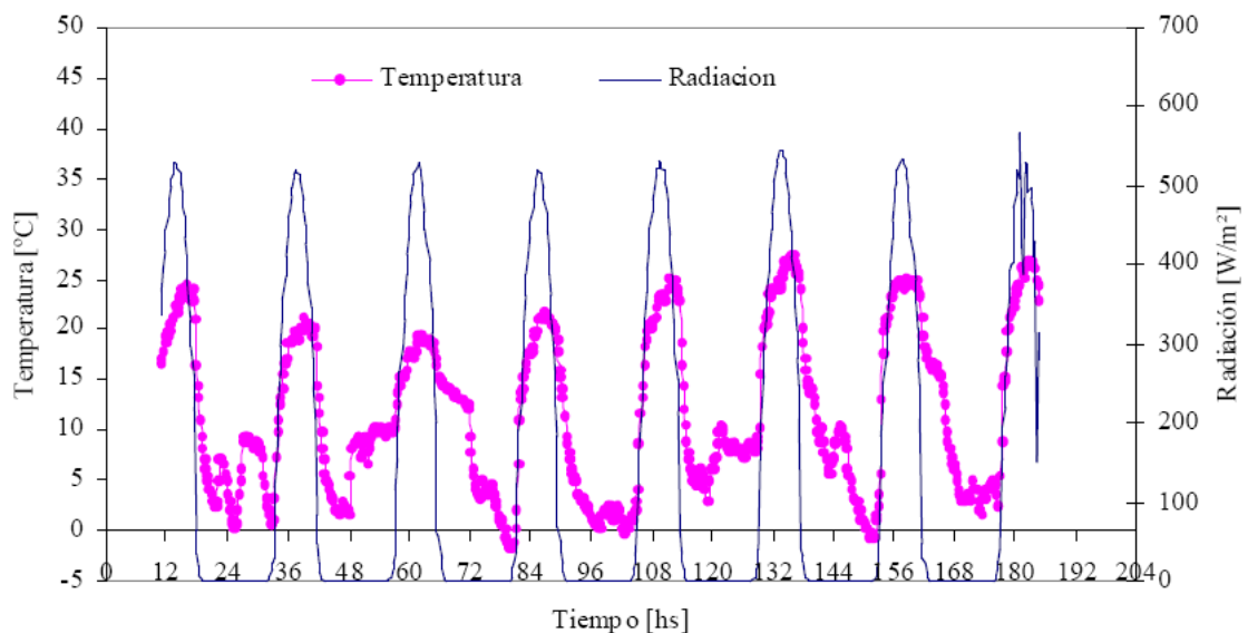
Fig. 14. Temperatura y radiación exterior.
