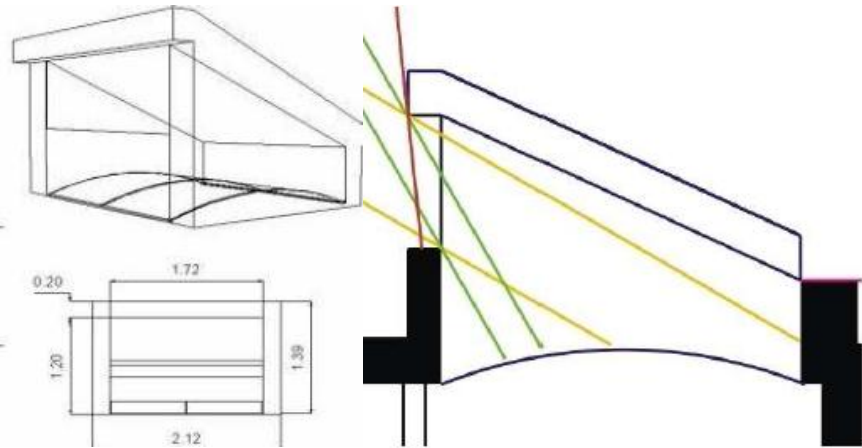
Fig. 8. Detalle del conjunto diseñado
